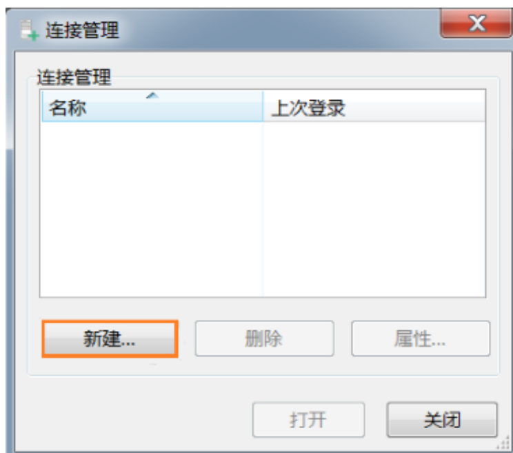
图2-3 连接管理
