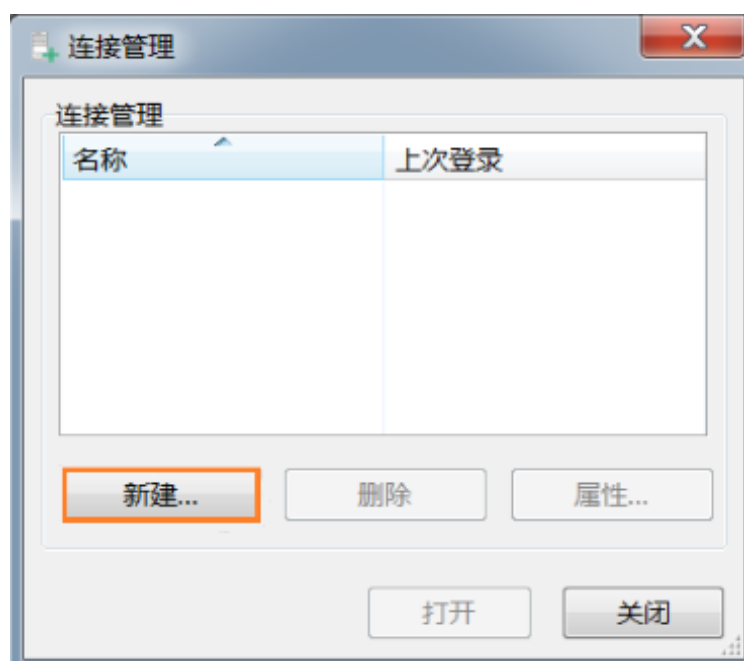
图2-7 连接管理
