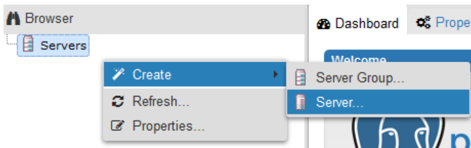
图6-1 创建
