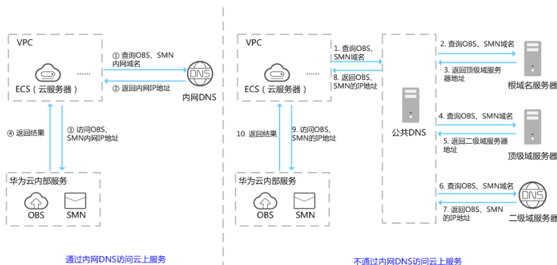
图1-3 访问华为云内部服务
