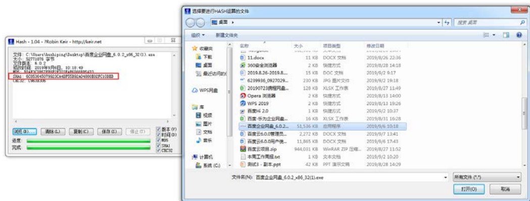
图 2.11-5 获取校验码
