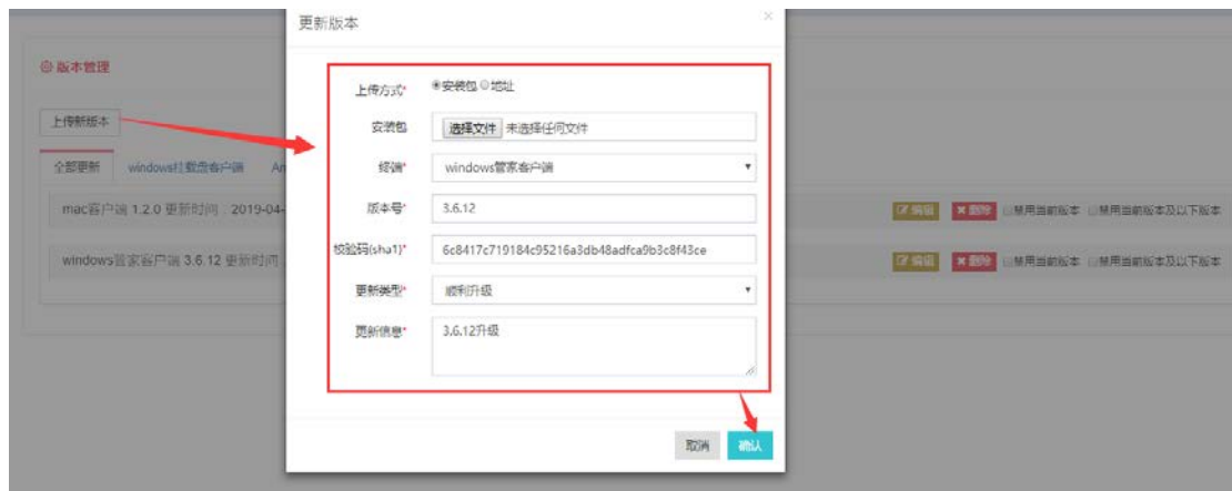
图 2.11-4 上传新版本
