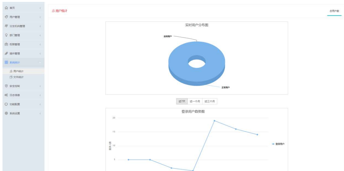
图 2.7-1 用户统计
