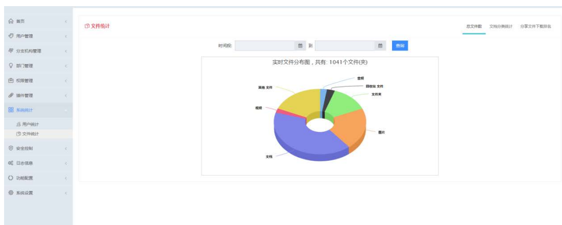
图 2.7-2 文件统计
