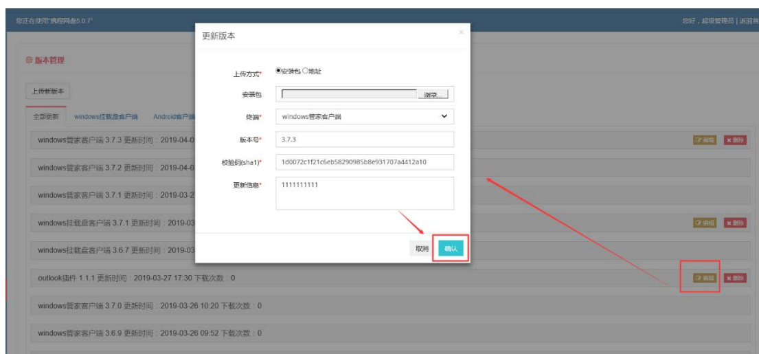
图 2.11-8 编辑版本
