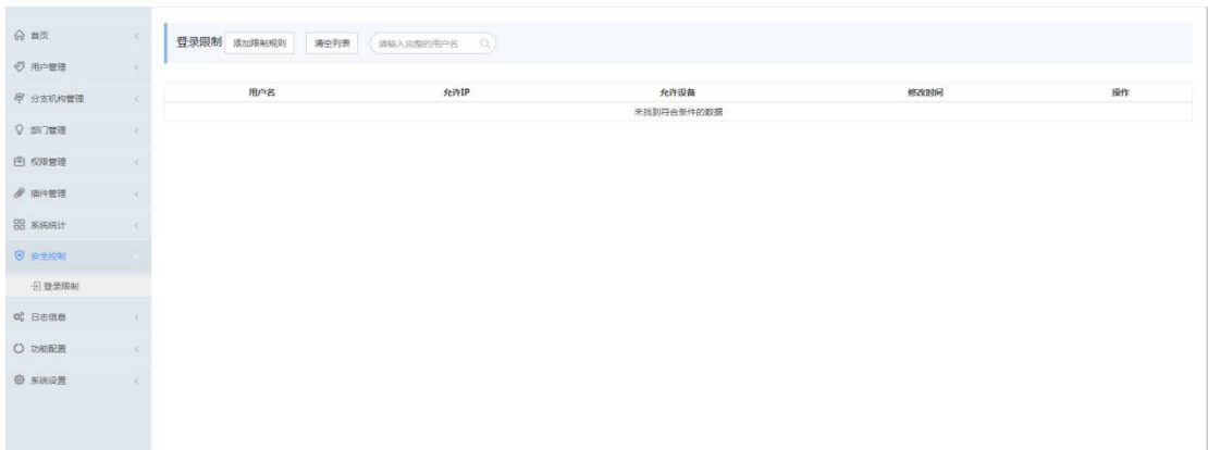
图 2.8-1 登录限制
