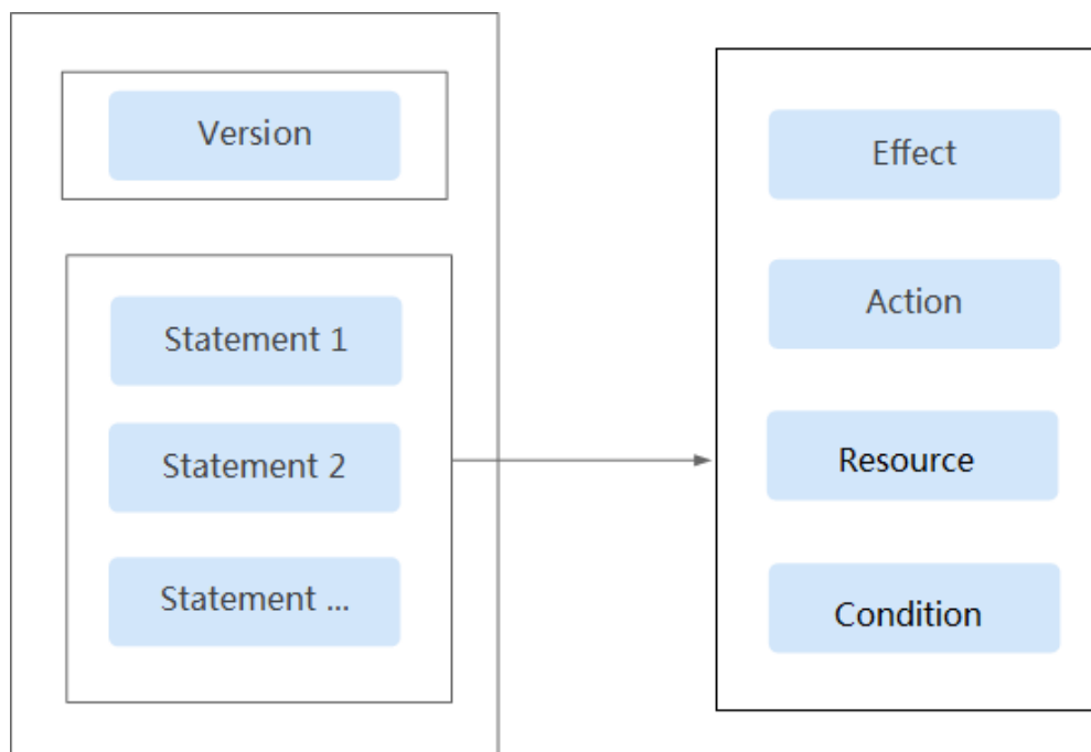
图4-1 策略结构
