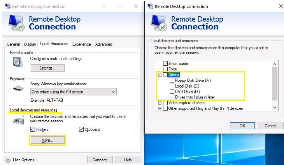
图 312 禁用 redirect local drives 功能
