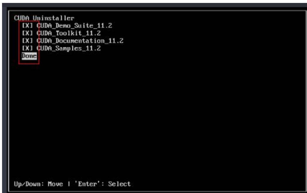
图 166 卸载 CUDA 驱动
