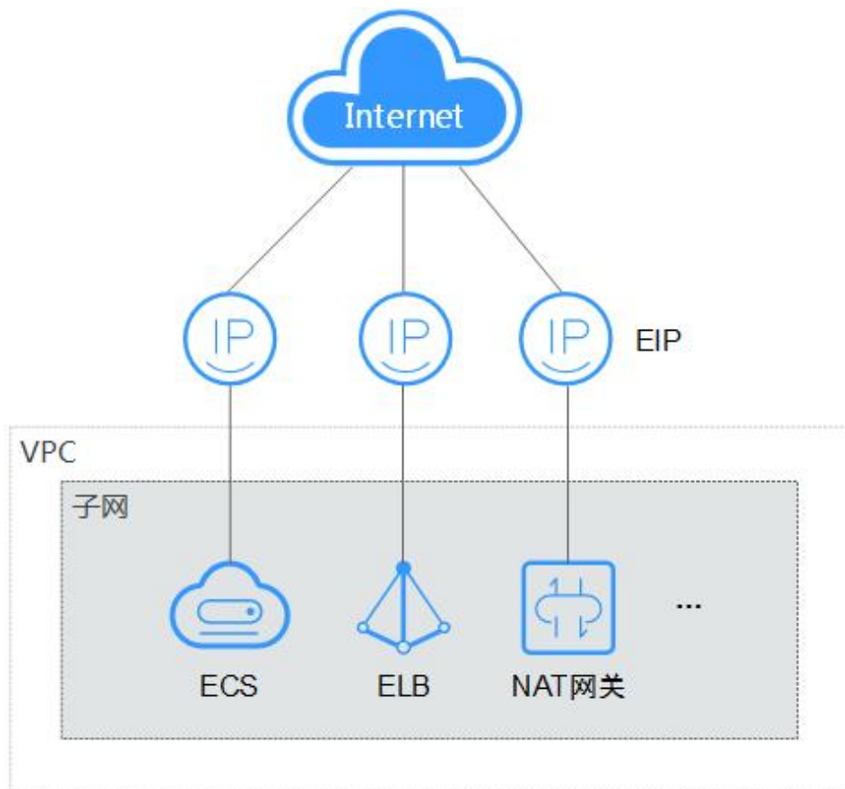
图 197 通过 EIP 访问公网
