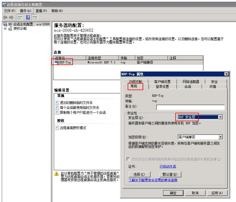
图 298 RDP-TCP 属性
