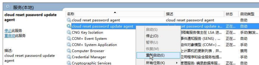
图 407 服务（本地）
