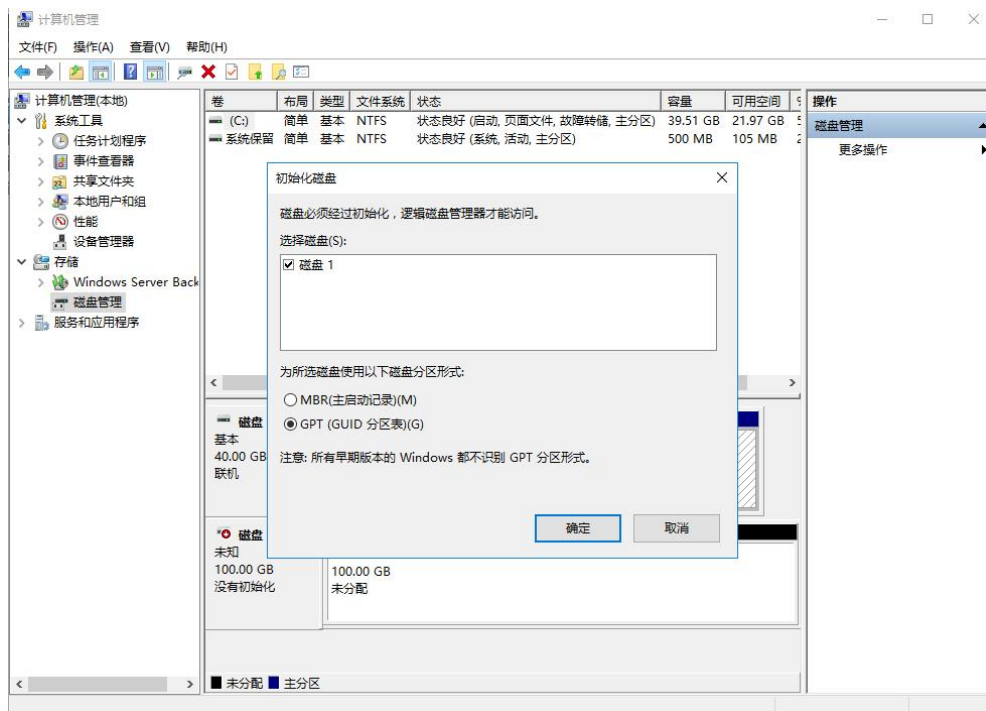
图 21 磁盘列表
