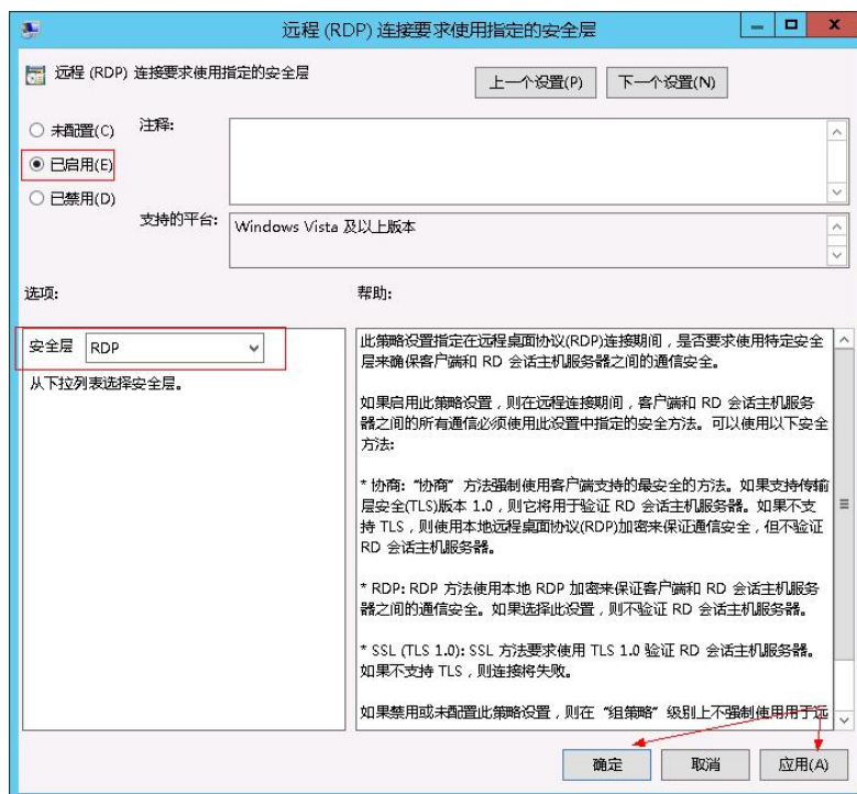
图 282 远程（RDP）连接要求使用指定的安全层
