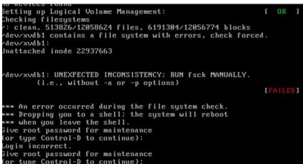
图 351 启动弹性云主机失败
