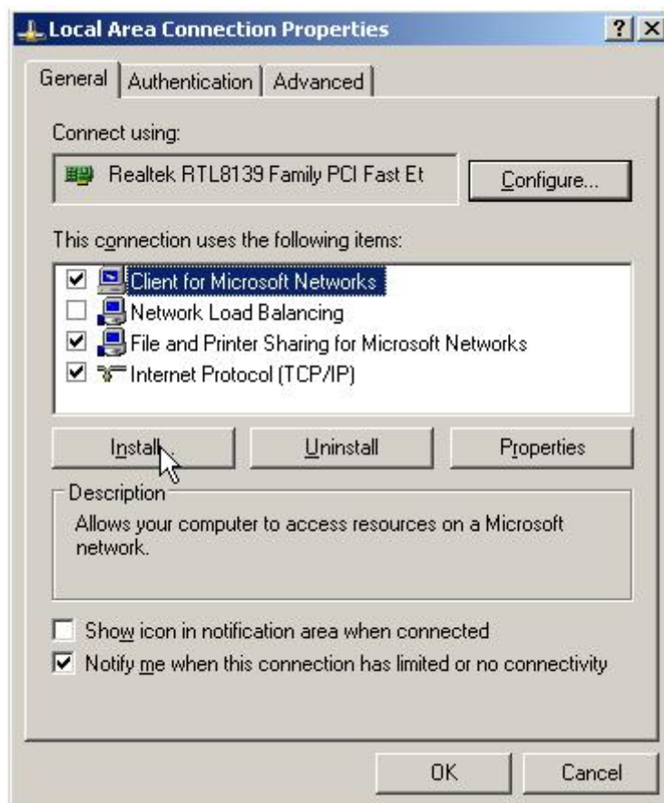
图 182 启用和配置 IPv6
