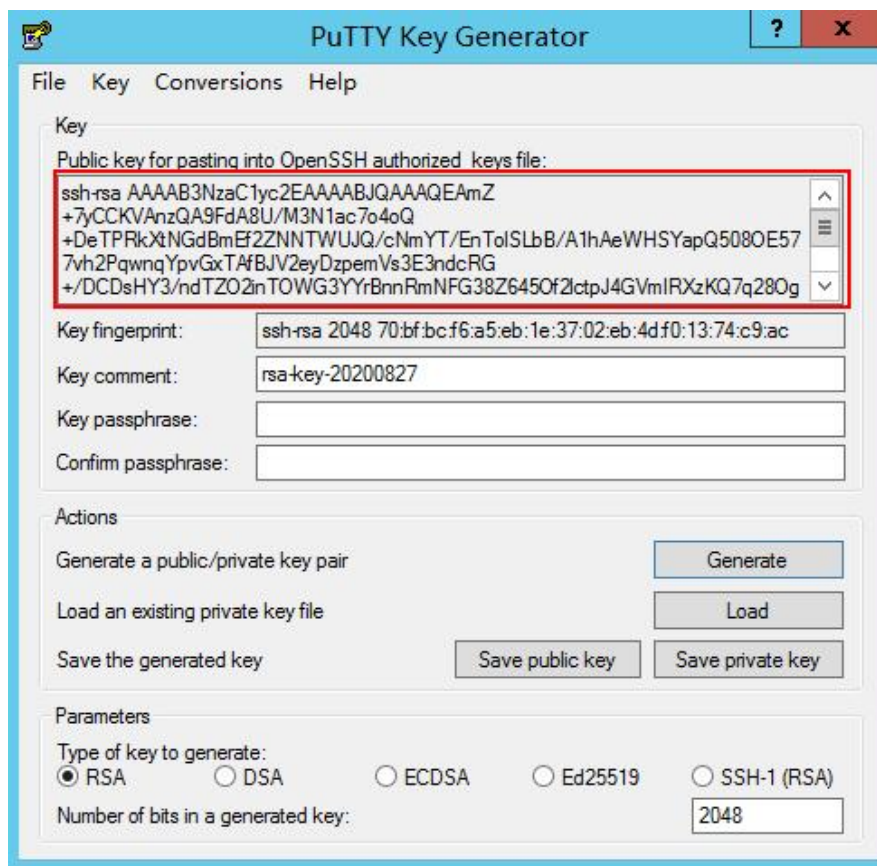
图 220 生成公钥和私钥文件
