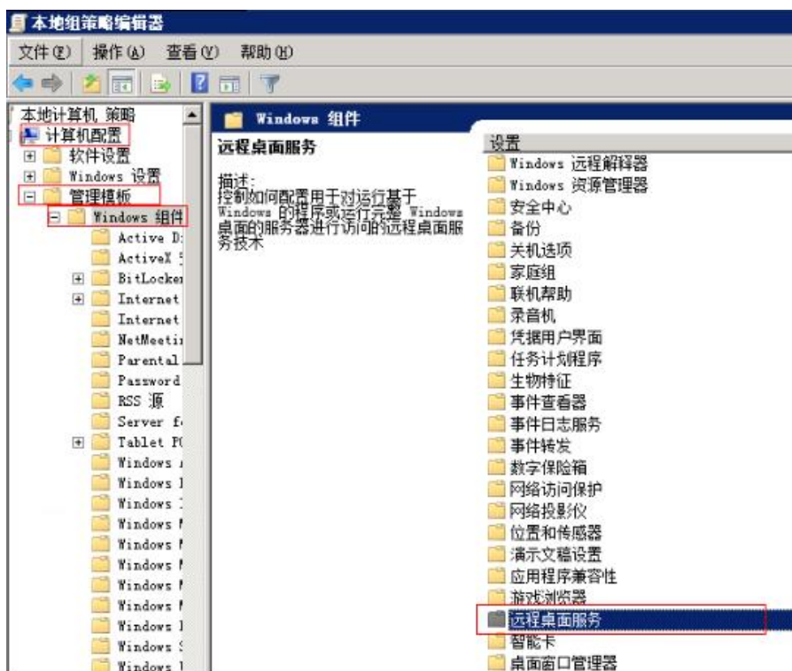
图 271 远程桌面服务
