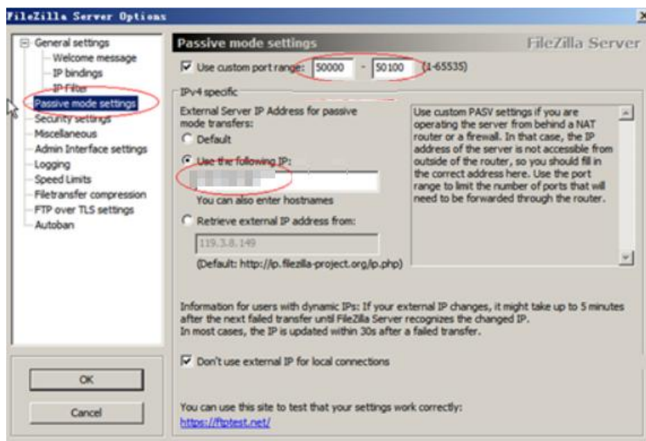
图 369 设置数据传输端口范围
