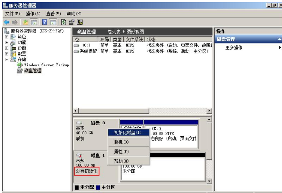
图 10 初始化磁盘
