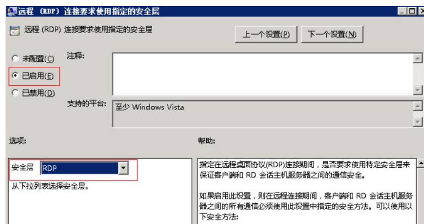
图 273 设置安全层
