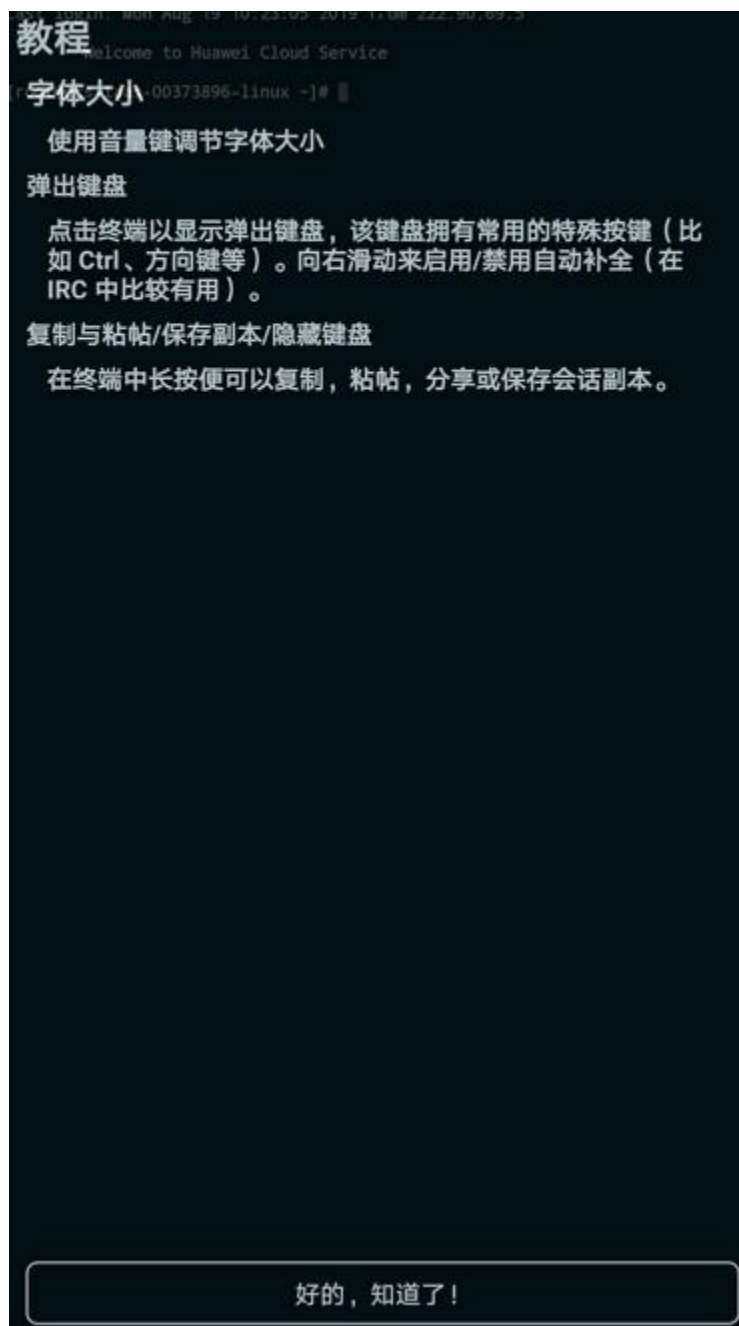
图 91 教程
