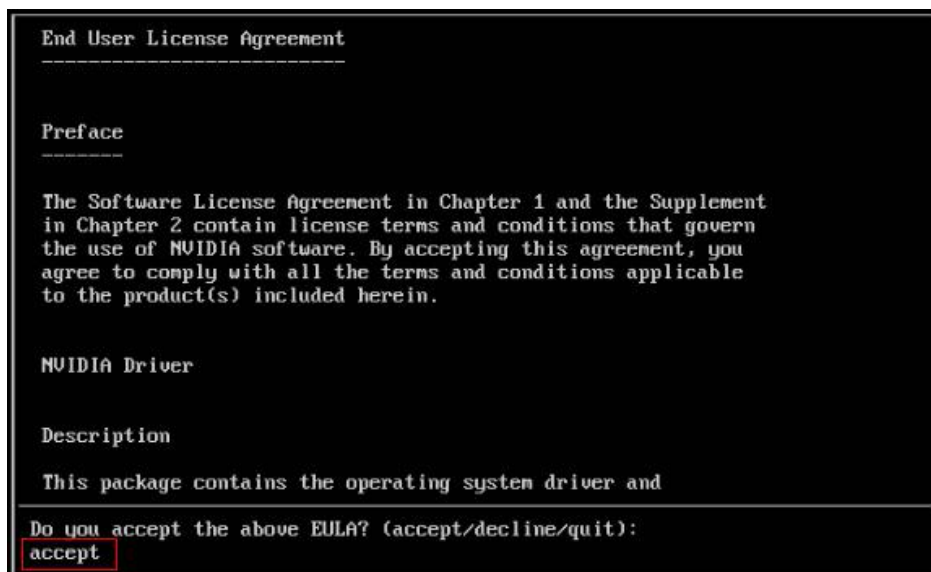
图 146 安装 CUDA_1
