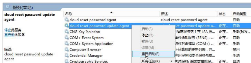
图 404 服务（本地）
