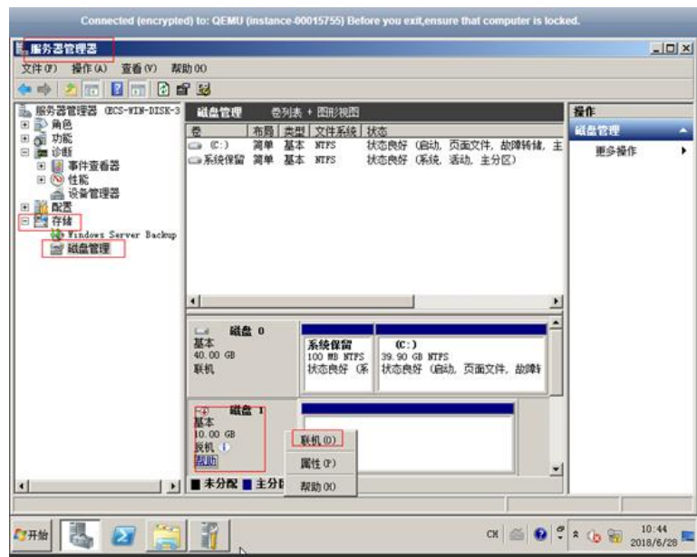
图 329 联机
