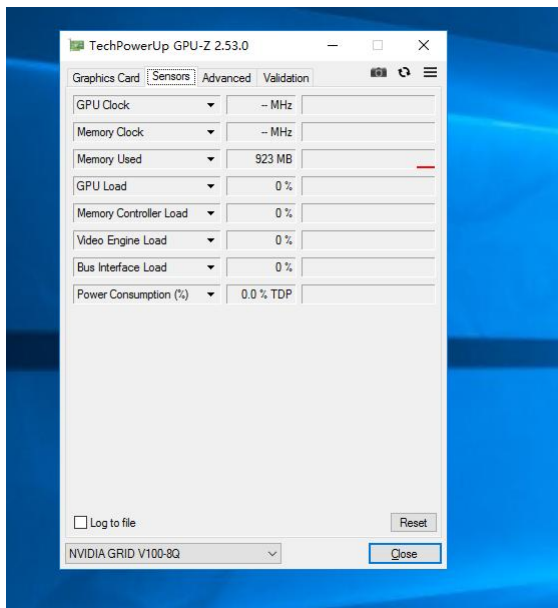
图 353 GPU 使用率
