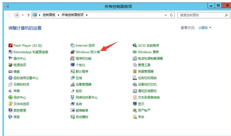
图 252 Windows 防火墙
